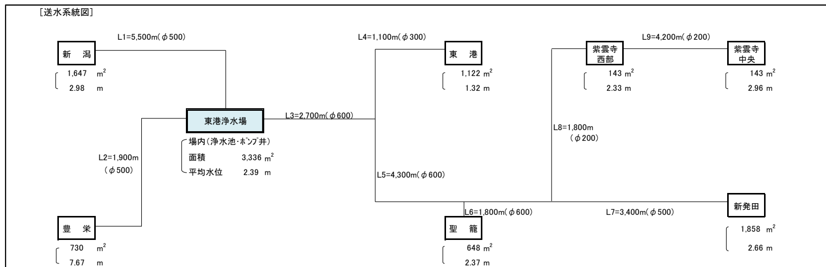
図 3 送水系統図
