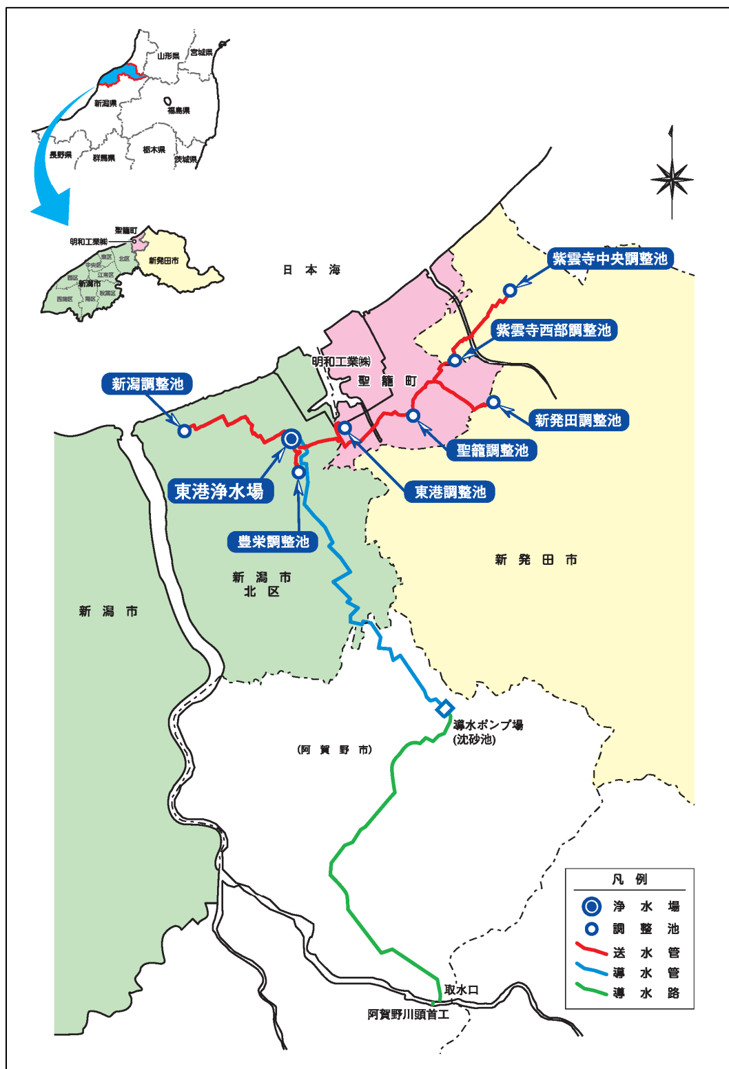
図 1 企業団管路図
