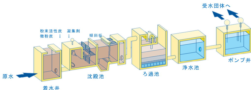
図2 浄水処理フロー
