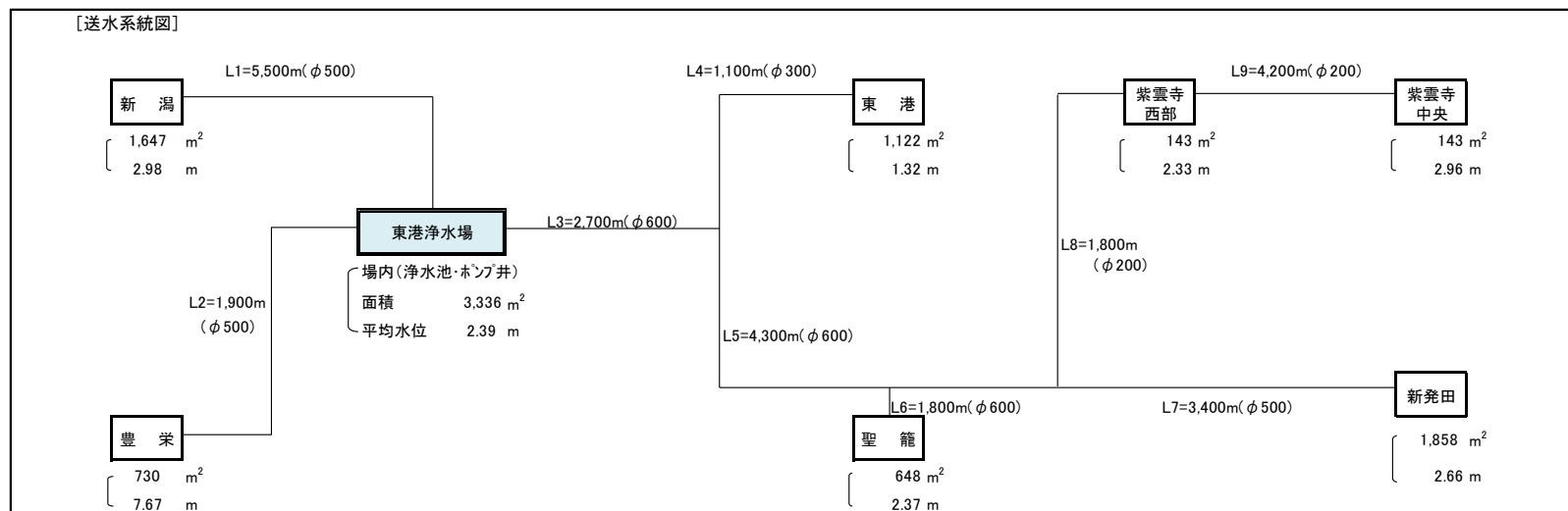
図 3 送水系統図
